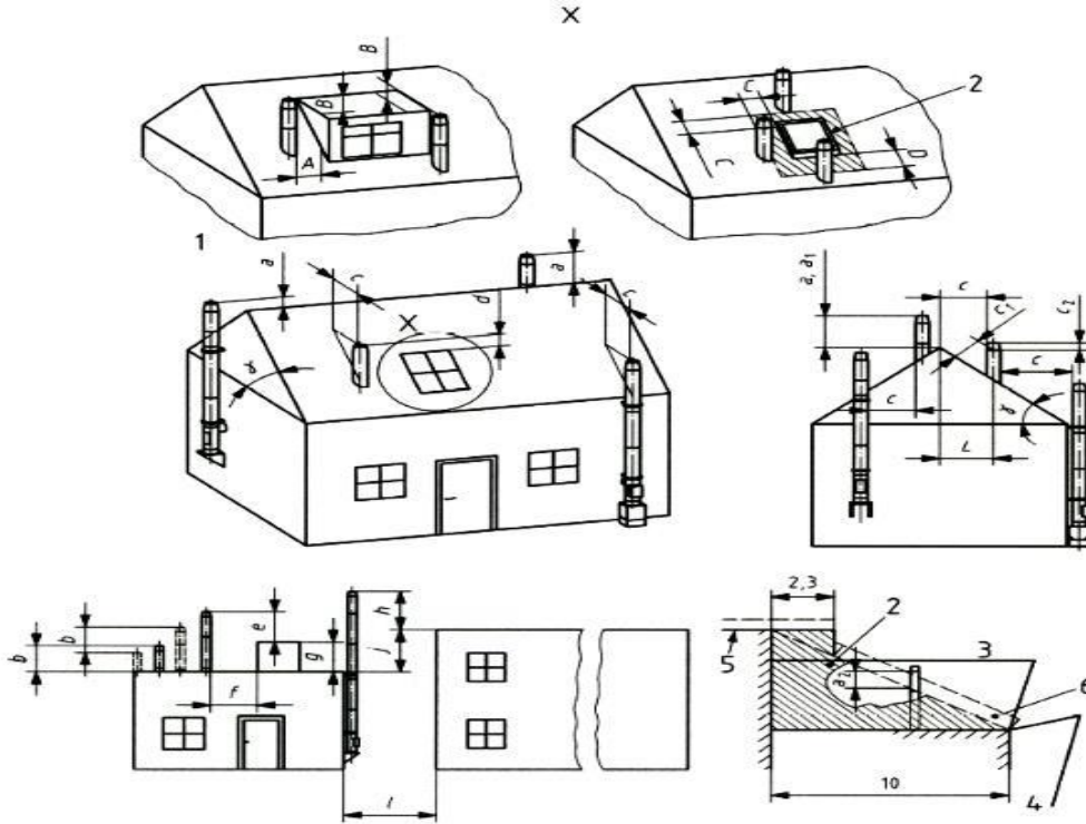
Şekil 17 – Baca çıkış konumu mesafeleri (bk. Tablo 9)
