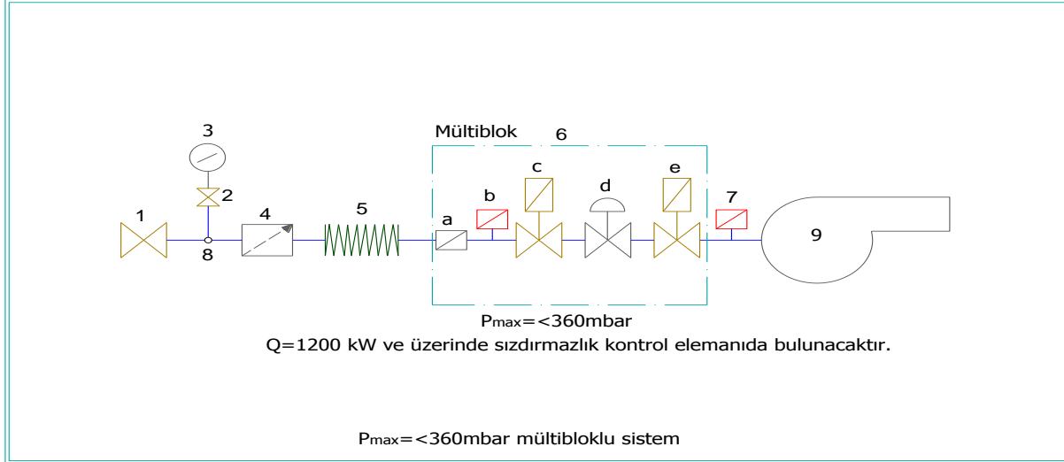
Şekil 28 - Multiblok brülör gaz kontrol hattı ekipmanları
