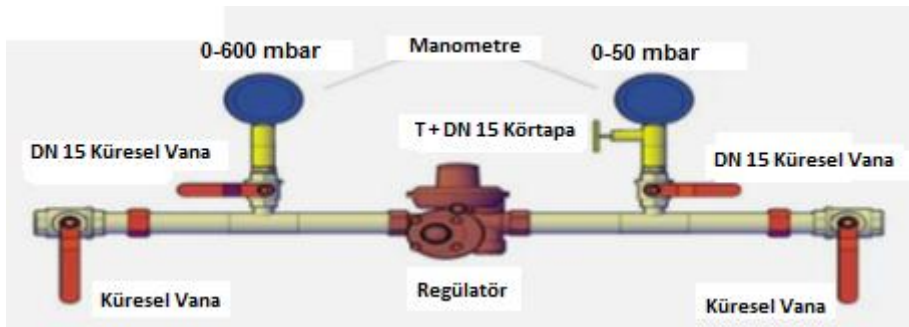
Şekil 13 – Regülatör Bağlantısı
