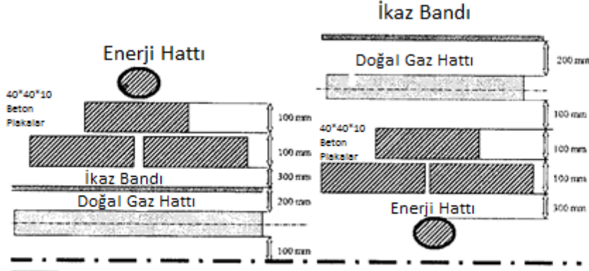
Şekil 4 – Doğal gaz hattı ile elektrik kabloları arasındaki mesafe
