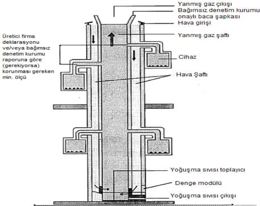
Şekil 31 -Hava-Atık gaz Bacası
