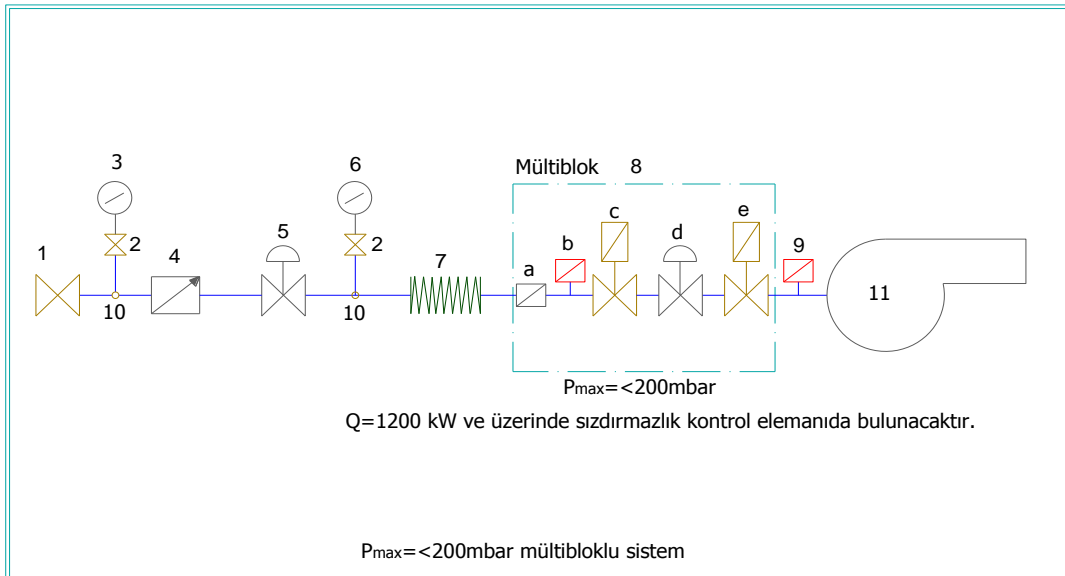
Şekil 29 - Multiblok brülör gaz kontrol hattı ekipmanları
