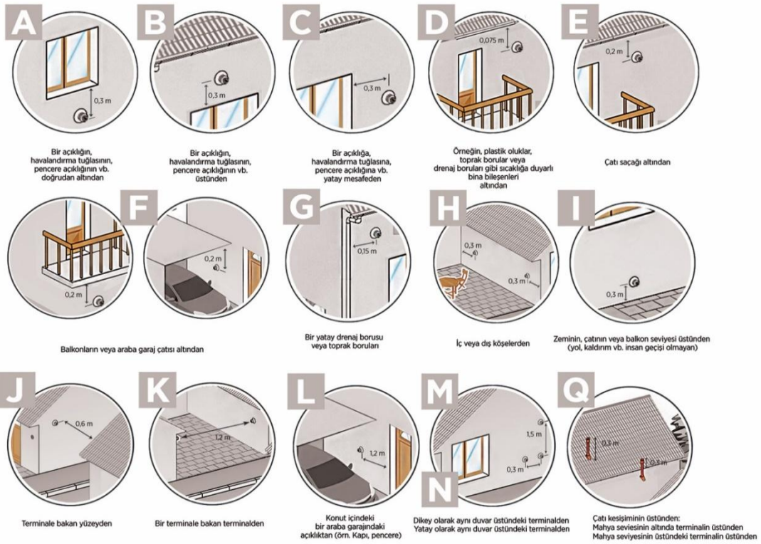
Şekil 18 – Denge duman yolu baca konfigürasyonları çıkışlarının konumu örneği
