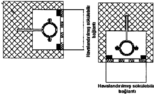
Şekil 9 - Siva üstü kanal içi boru kelepçesi
